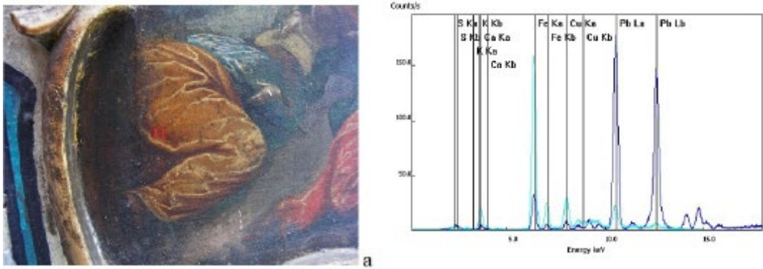
Fig. 7. Icoana Schimbarea la Față a. Proba 11 pigment galben - brun veșmânt Sf. Petru; b. Spectrul XRF pigment brun
